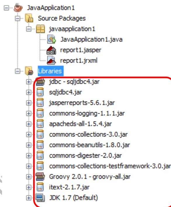
Hình 10 – Các thư viện (file .jar) cần thêm vào ứng dụng Java
