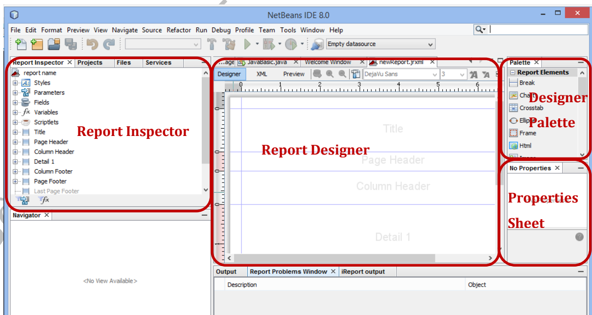
Hình 4 – Giao diện iReport
